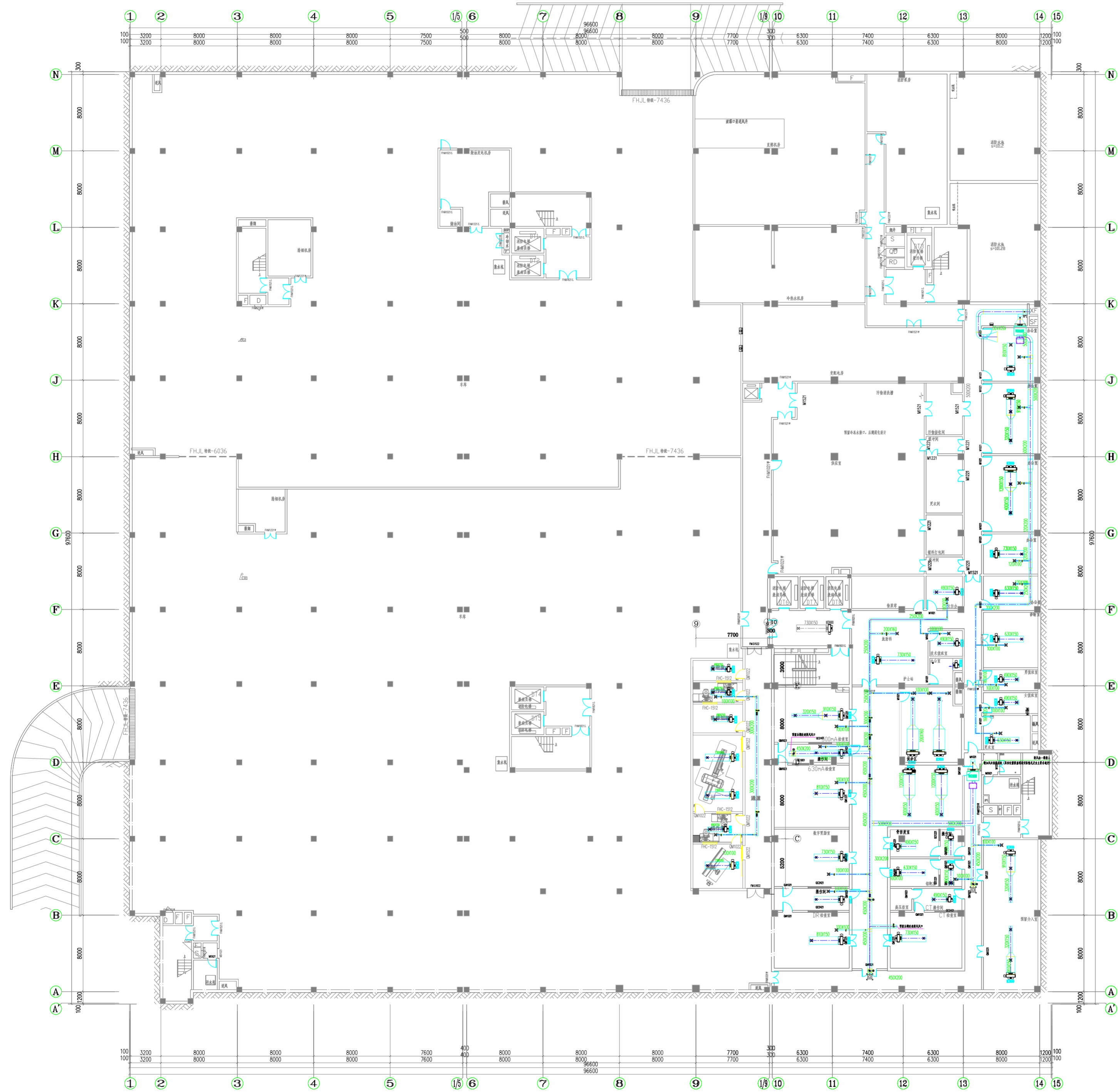
负一层业务用房区域新风整改平面布置图
